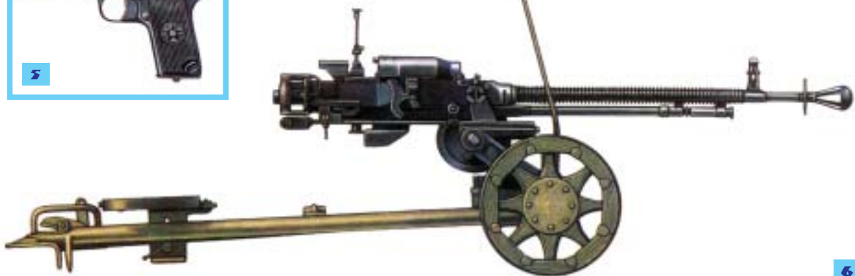
Стрелковое оружие Красной Армии: 1. 7,62-мм ручной пулемет образца 1927 г. (ДП). 2. 7,63-мм пистолет-пулемет образца 1941 г. (ППШ). 3. 7,62-мм пистолет-пулемет образца 1943 г. (ППС). 4. 7,62-мм револьвер системы Нагана образца 1895 г. 5. 7,62-мм пистолет образца 1930 г. (ТТ). 6. 12,7-мм крупнокалиберный пулемет образца 1938 г. (ДШК).
